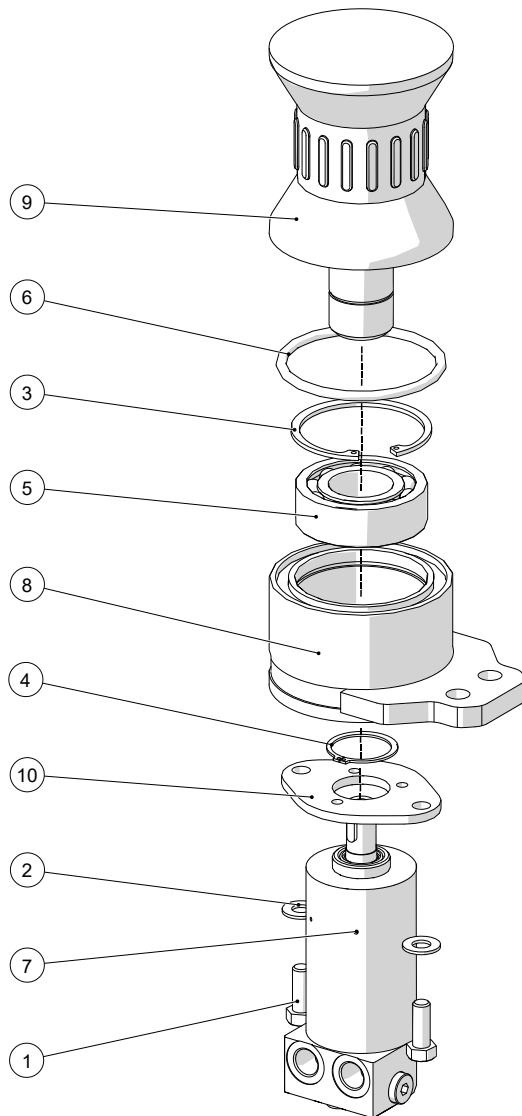
205.121.000 Conjunto rodillo axial L
